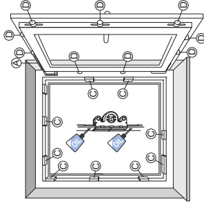
Bild 1: Schmierstellenübersicht
