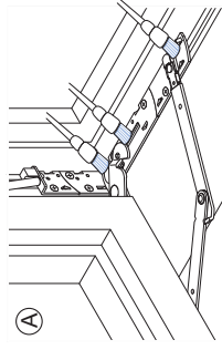
Bild 3: Ecklager
